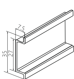
TH35x7,5
